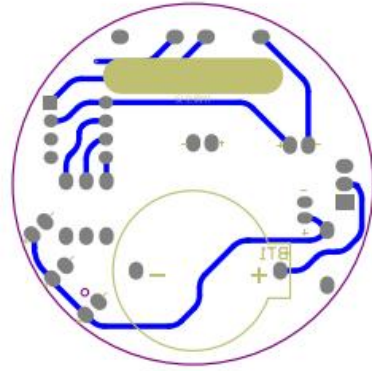
PCB 反面
